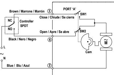
Abb. 9: VC-Stellglied für SPDT-Regler
